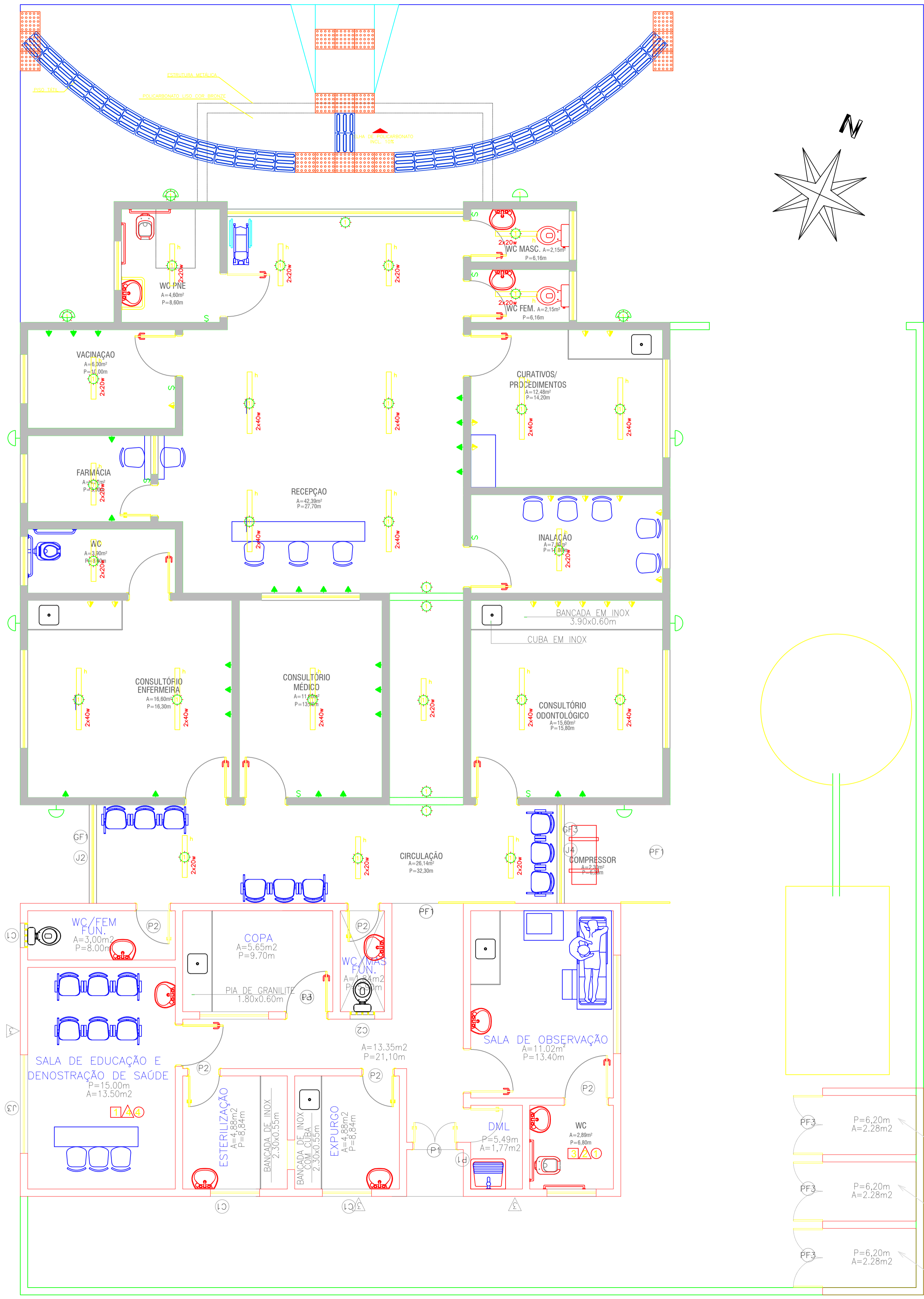
DISTRIBUIÇÃO DE LUMINARIAS E PONTOS ESCALA 1/50
