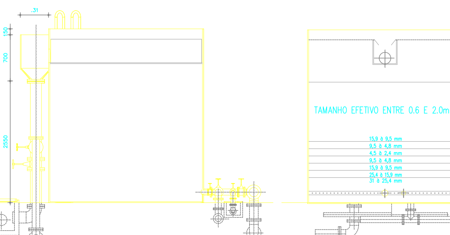
CORTE DD ESCALA 1:40
