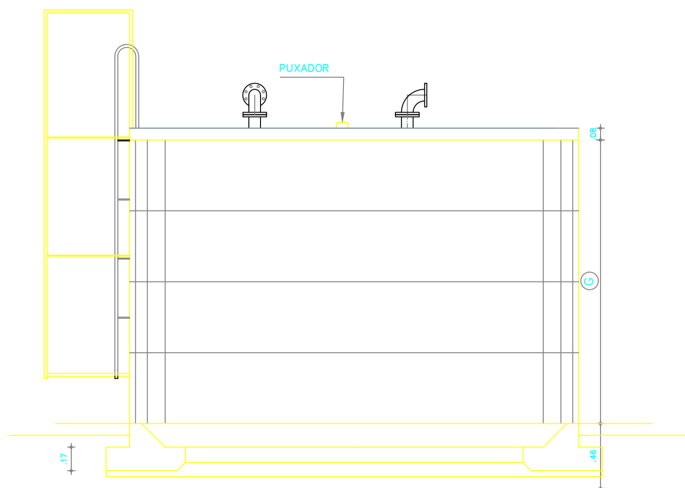
VISTA FRONTAL ESCALA 1:40
