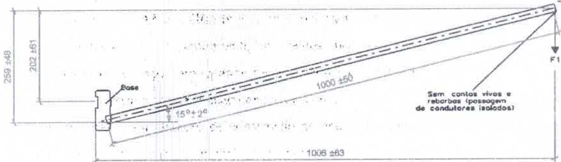
Figura 17 – Braço padrão COPEL tipo BR-1.
