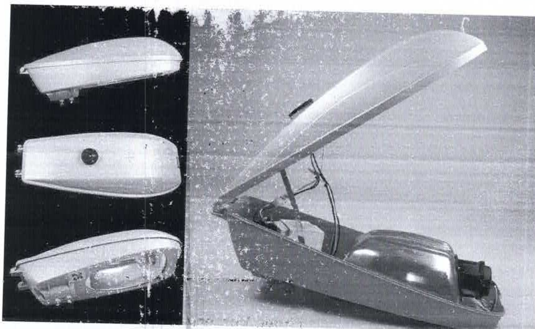
Figura 16 - Exemplos de uma luminária integrada. Fonte: COPEL (2012).
