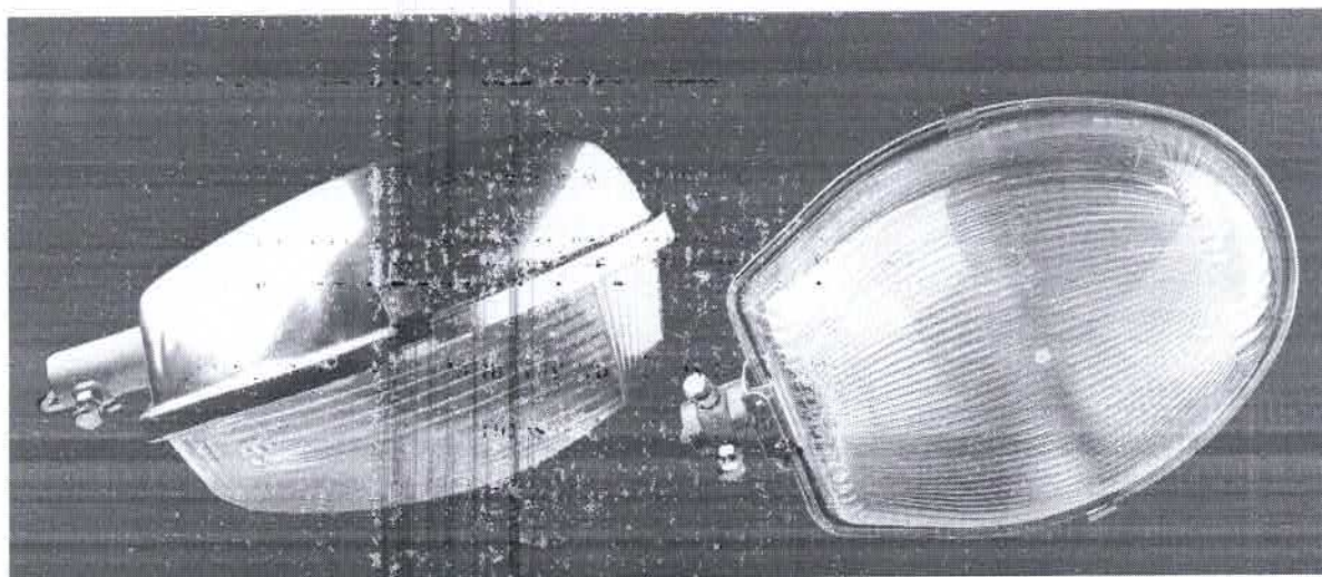
Figura 15 – Um modelo de luminária fechada sem equipamento.
