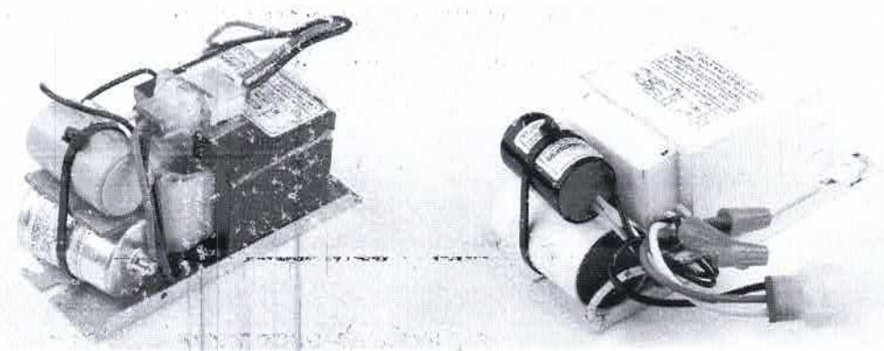
Figura 10 – Reator interno.
