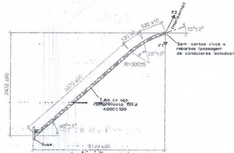
Figura 19 -- Braço padrão COPEL tipo BR-3.
