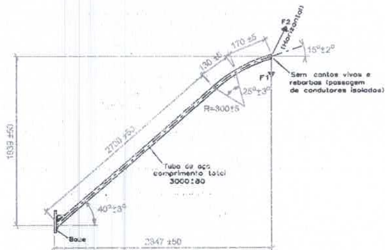
Figura 18 – Braço padrão COPEL tipo BR-2.
